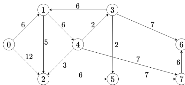
Figure 7.2 – Problème de flot maximum
