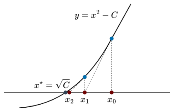
Figure 5.1 – Exemple de méthode de Newton
